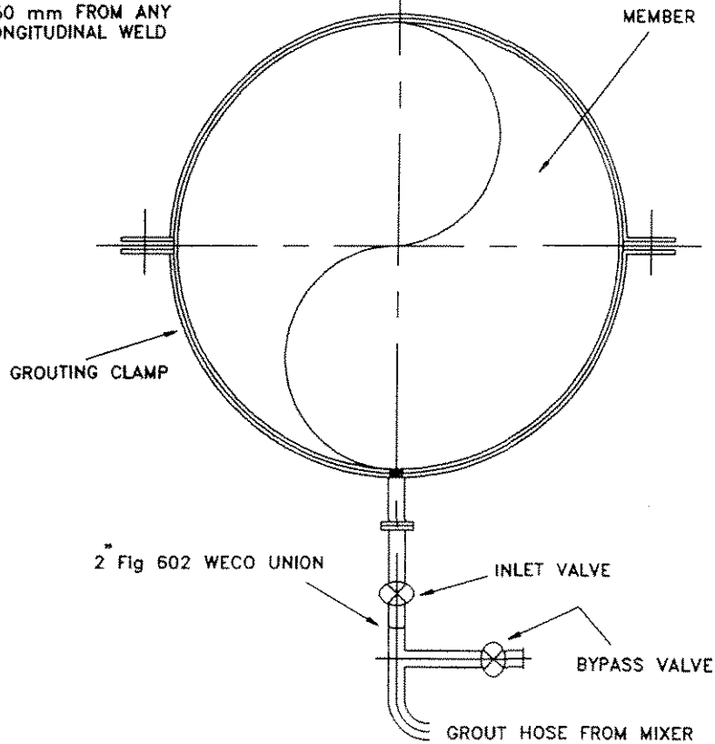
VIEW A-A
